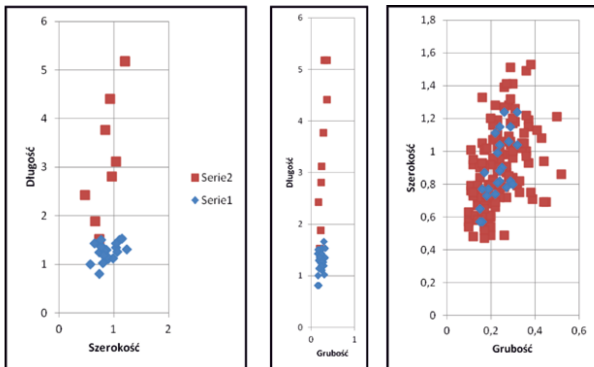
Ryc. 144. Redecz Krukowy, stan. 20. Graficzne odwzorowanie parametrów wiórów i rylców z skupienia 2. Kolor czerwony – wióry; kolor niebieski – rylcowce.
