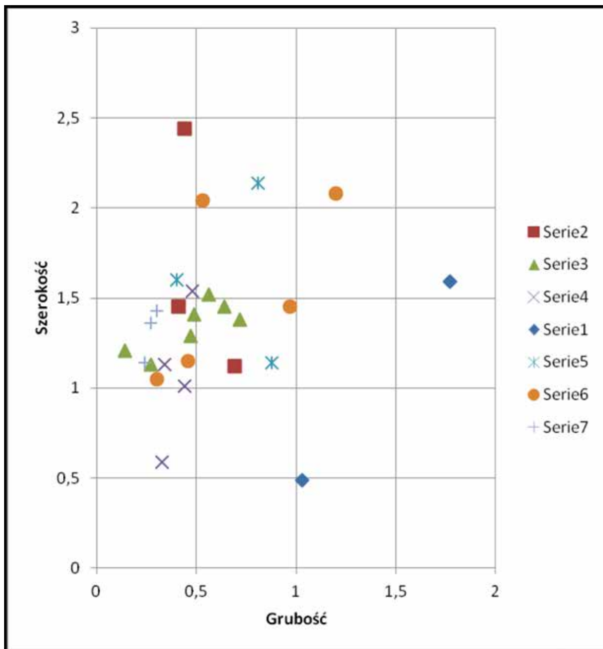
Ryc. 145. Redecz Krukowy, stan. 20. Graficzne odwzorowanie parametrów narzędzi ze skupienia 2. 1 – drapacze; 2 – fragment odłupka; 3 – odłupki retuszowane; 4 – przekłuwacze; 5 – skrobacze; 6 – skrobacze z pazurem; 7 – wióry retuszowane.
