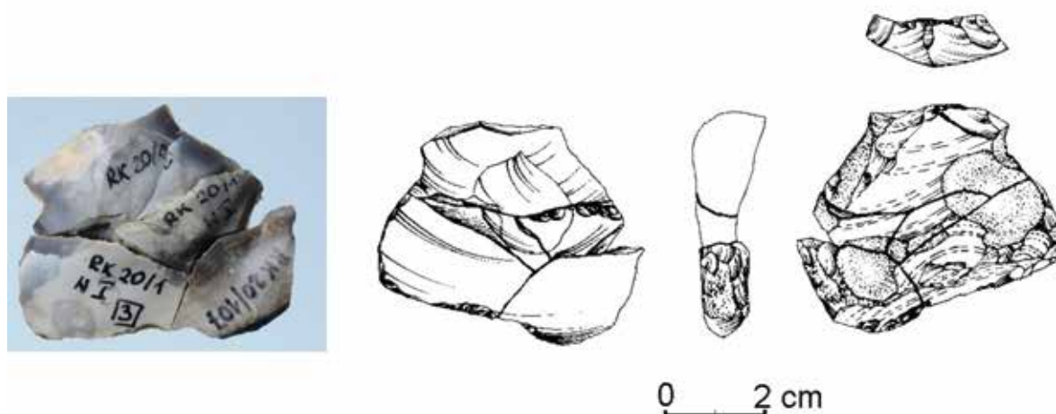
Ryc. 139. Redecz Krukowy, stan. 20. Składanka narzędzi ze skupienia 1.
